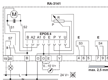
比例控制型接线图
