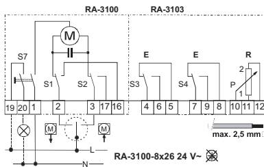
3 线控制型接线图
